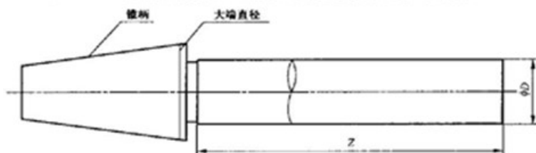
图 A.1 检验芯轴
