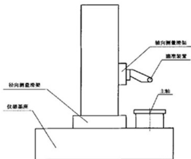
图1 刀调仪的型式与主要部分名称
